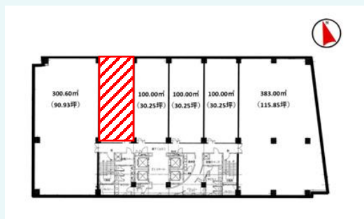
5階平面図
