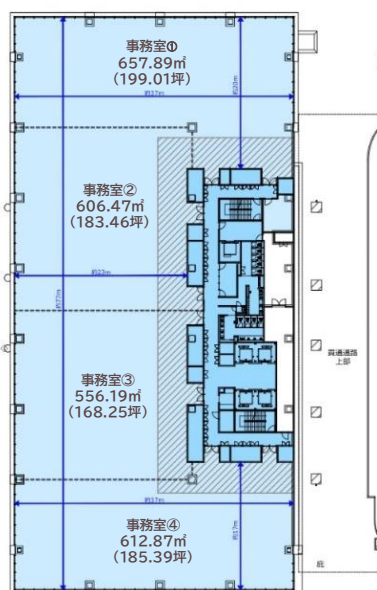
■ 基準階(3階～5階)平面図
