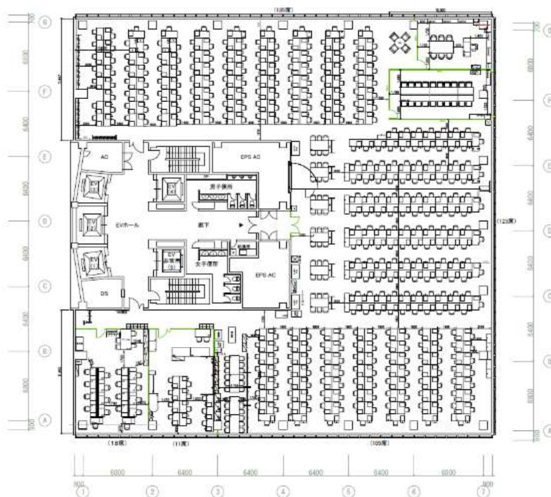
12階 現行レイアウト図
